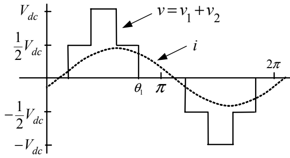
Fig. 2. Output waveform
